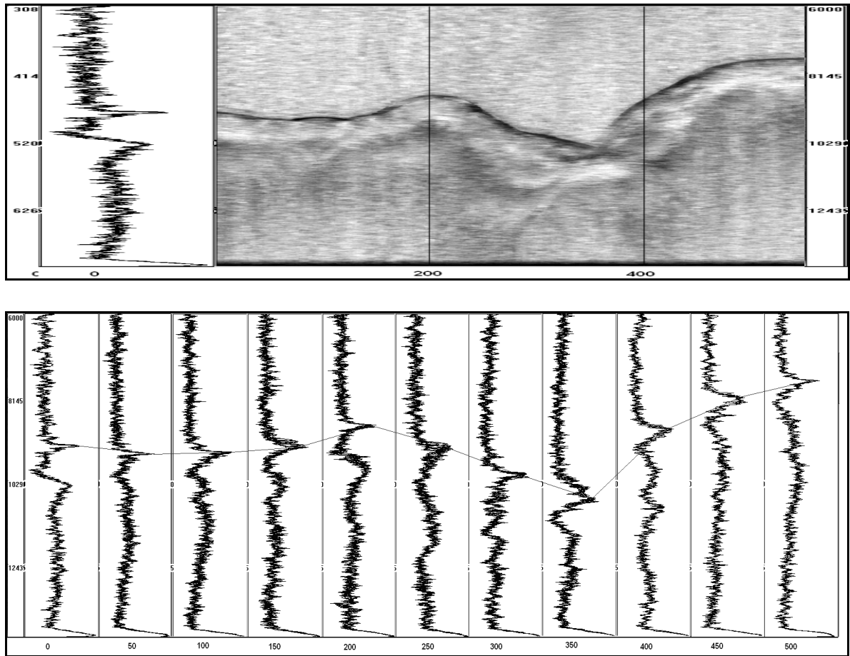
Рис. 5.1. Развертка приращения фазы (частоты) отраженного сигнала и профиль изменения для первой строки (сверху). Снизу профили частоты для отдельных строк, начиная со строки 0 с шагом в 50 строк. Усреднение при обработке частоты по 9 строкам, и 21 отсчету. Ломаная линия на нижней части соответствует линии дна.
