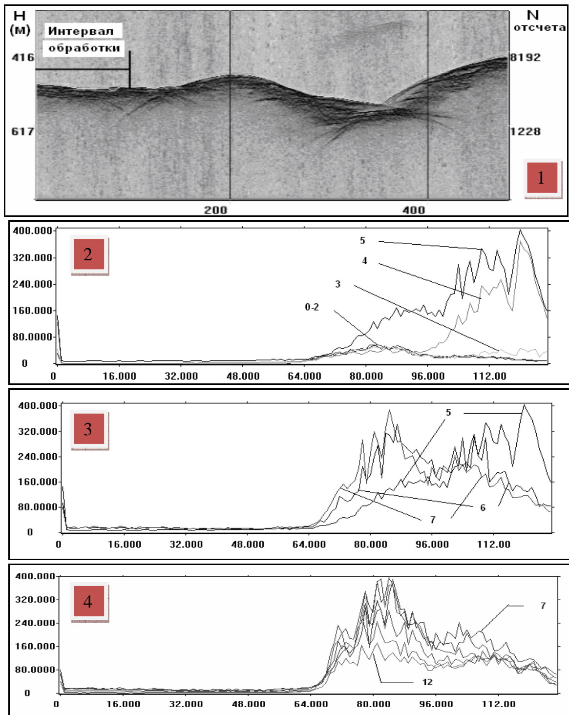
Рис. 3. Акустическое изображение (1) и последовательное изменение спектра сигнала (2,3,4). По оси абсцисс указан номер спектрального отсчета, пропорциональный частоте.
