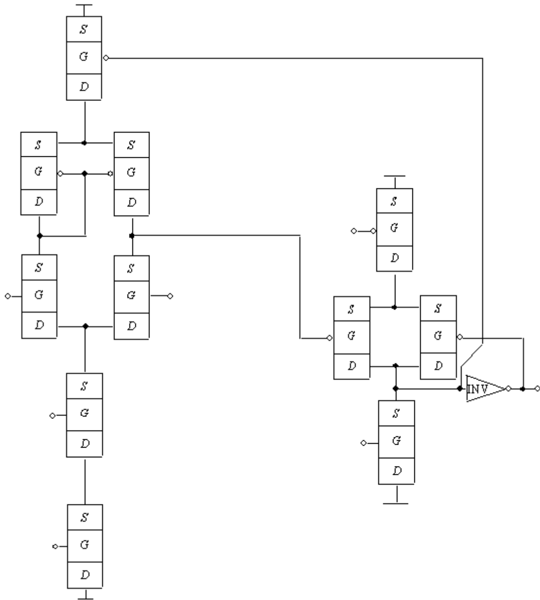
Рис. 1. Схема рассматриваемого компаратора [4]
