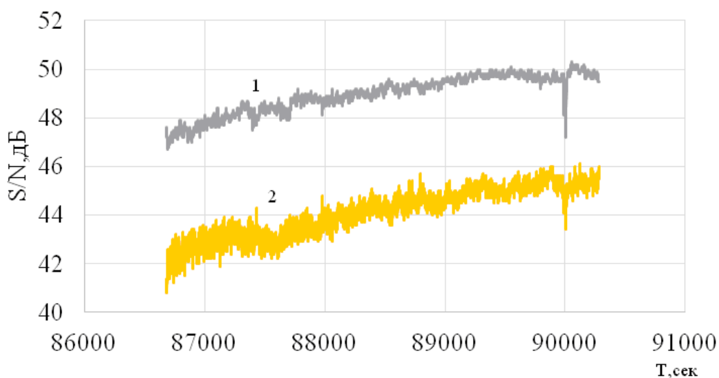
Рис.2. Кривые отношения сигнал/помеха, полученные при обработке сигналов глобальной спутниковой навигационной системы GPS: 1 – центральная частота f = 1575 МГц; 2 – центральная частота f = 1227 МГц (обработано в ФИРЭ им. В.А.Котельникова РАН).
